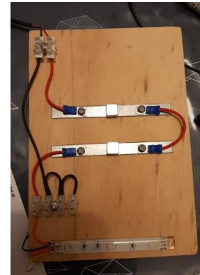
15 prototype af knapmekanisme
